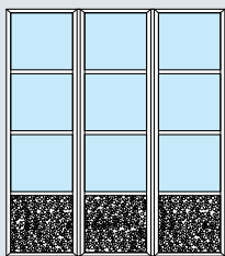
Wypełnienie PU, Aluminium przetłaczane w strukturze stucco 26 mm z przeszkleciem z tworzywa sztucznego 26 mm
