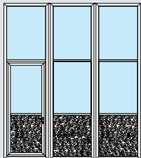
Wypełnienie PU, aluminium przetłaczane w strukturze stucco 26 mm z przeszkleciem częściowym
